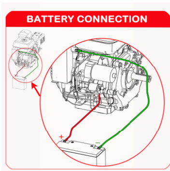
Batterie anschließen
