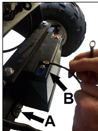
Batteriehalter montieren & Batterie anschließen
