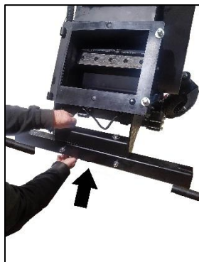
Hinterachse montieren
