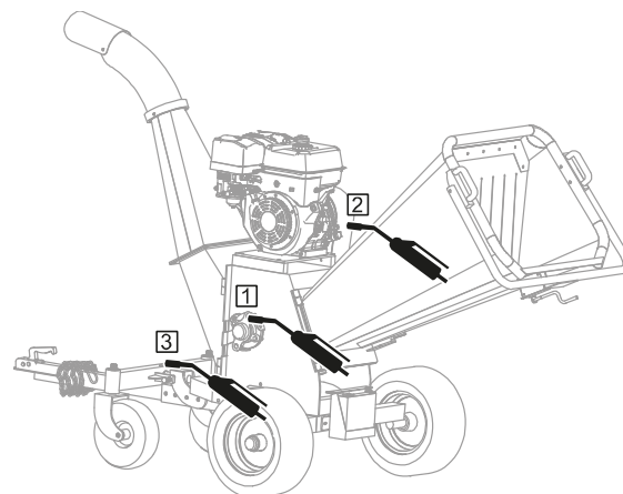
Schmierstellen Trommelhackwerk, Pendelachse
