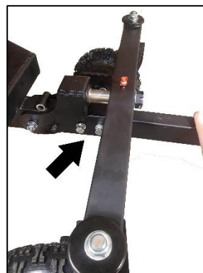
Zugstange montieren
