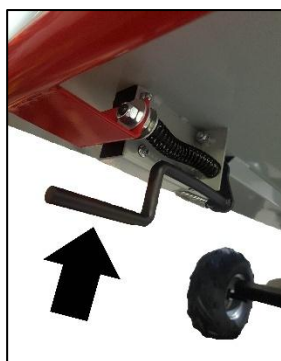
Not-Halt-Bügel unten
