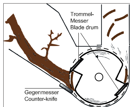
Trommelhackwerk
