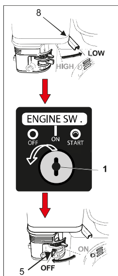
Motor abstellen
